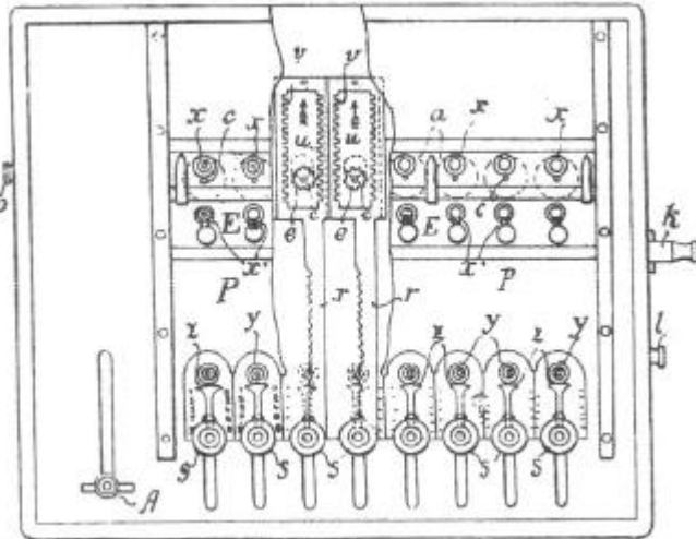
Abb. 3 Rechenwerk der „Adsumudi“: die patentierten Doppelzahnstangen (angetrieben durch den Schieber „A“) sorgen bei ihrer Abwärtsbewegung für Plus- oder Minusdrehungen der Zählräder „e“, je nachdem, ob das Zählwerk „E“ nach rechts oder links verschoben wird. Für Subtraktionen wird der Schieber „A“ ein wenig verdreht.
